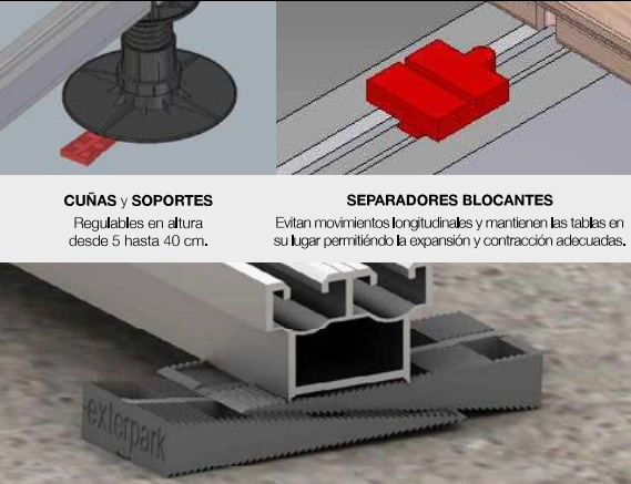
Rastrel con CUÑAS DENTADAS desde 1 hasta 50mm Rastrel en punta que ancla perfectamente en las cuñas para un nivelado adecuado.
