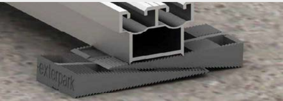
Rastrel con CUÑAS DENTADAS desde 1 hasta 50mm Rastrel en punta que ancla perfectamente en las cuñas para un nivelado adecuado.
